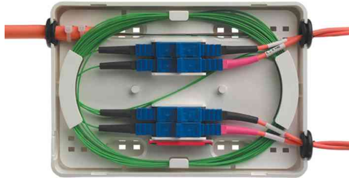
Symbolbild! Spleißbox mit 2 x SC-Duplex Kupplungen und Faserpigtails
